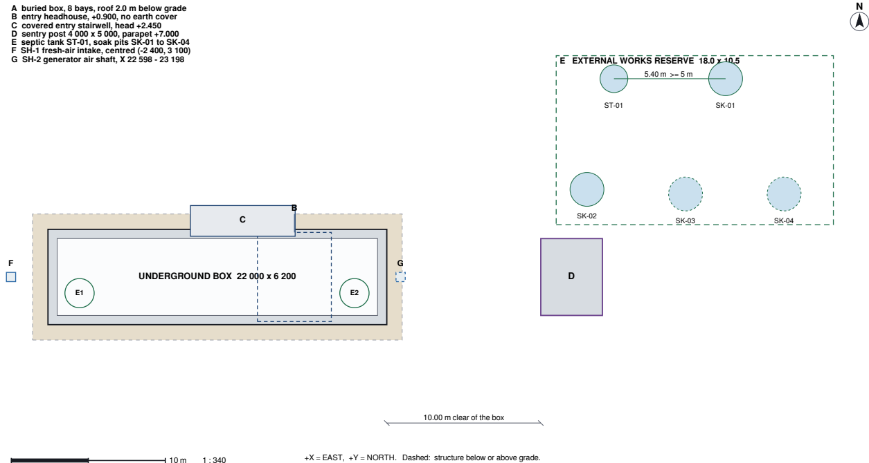
Fig 2.6 : Site Layout Plan
