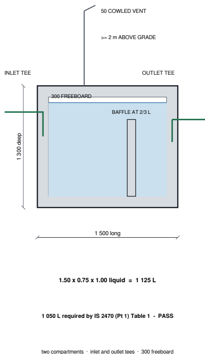
ST-01 SEPTIC TANK 1 : 40
