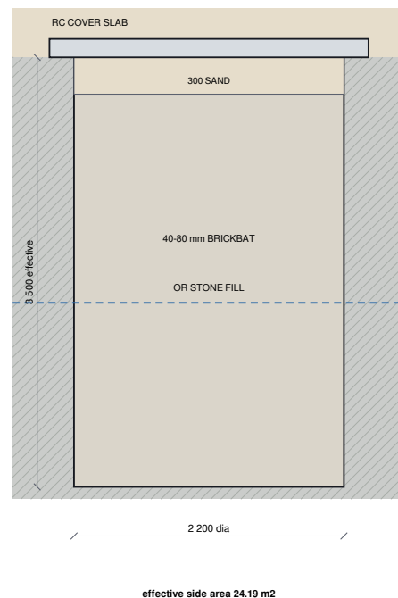
SK-01 / SK-02 SOAK PIT 1 : 55
