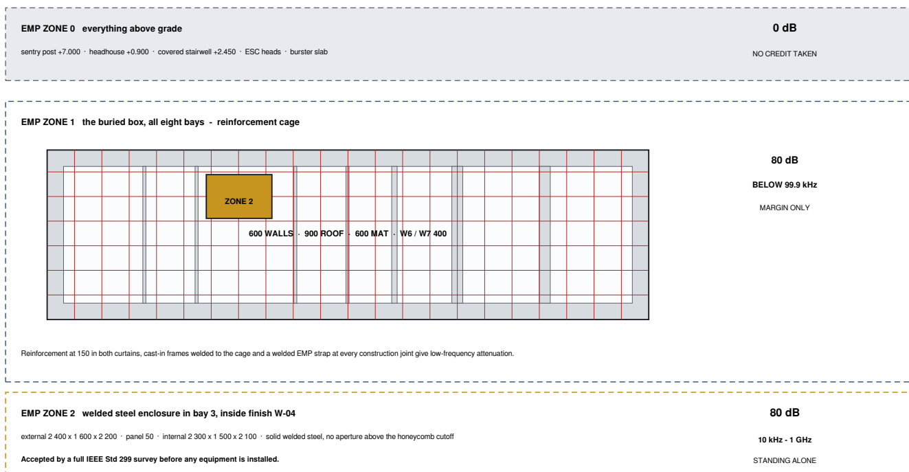
Fig 11.1 : EMP Zones
